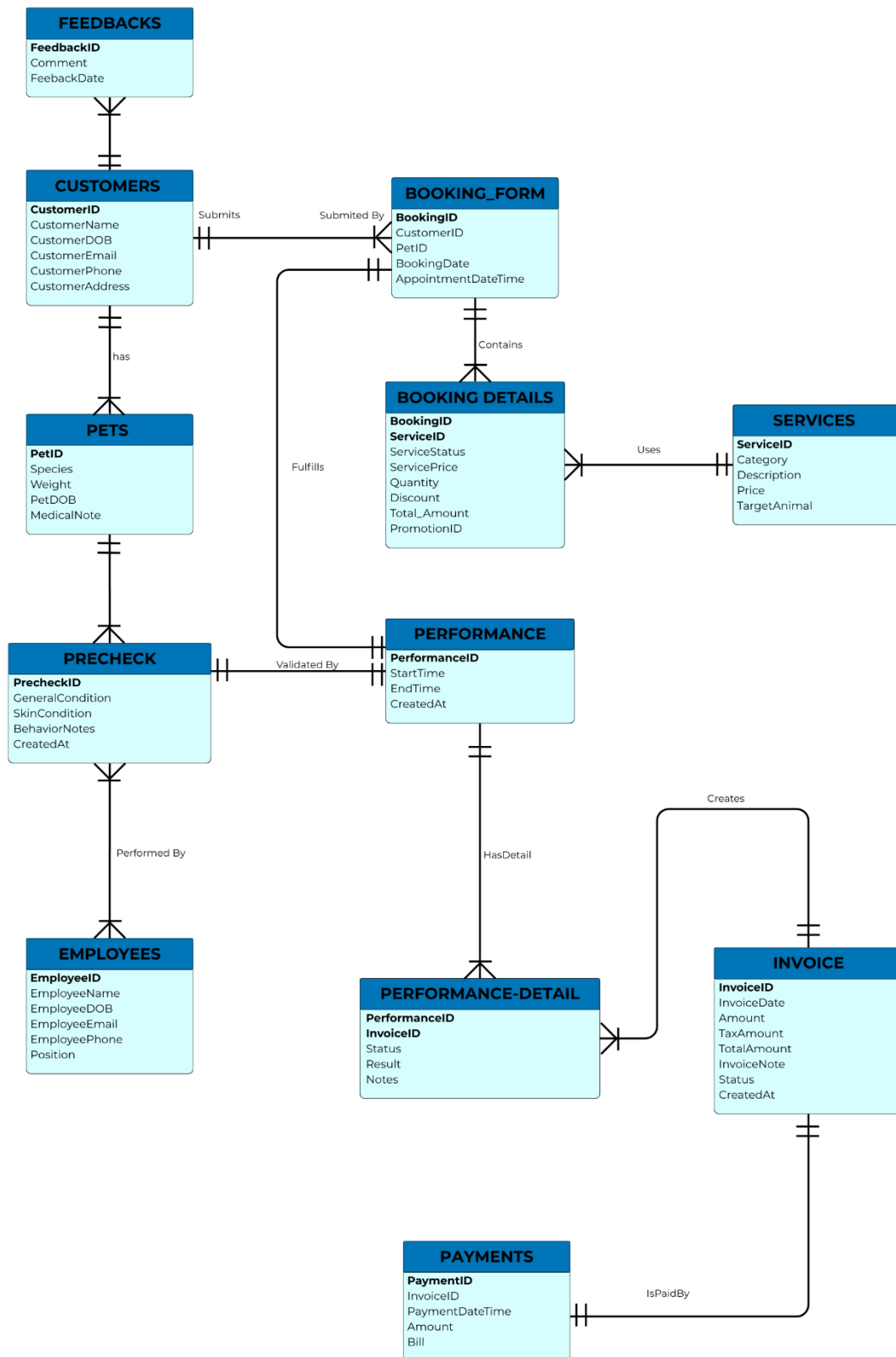
Hình 1: Sơ đồ mô tả mối quan hệ thực thể ER (hoặc ERR) của UrPet
